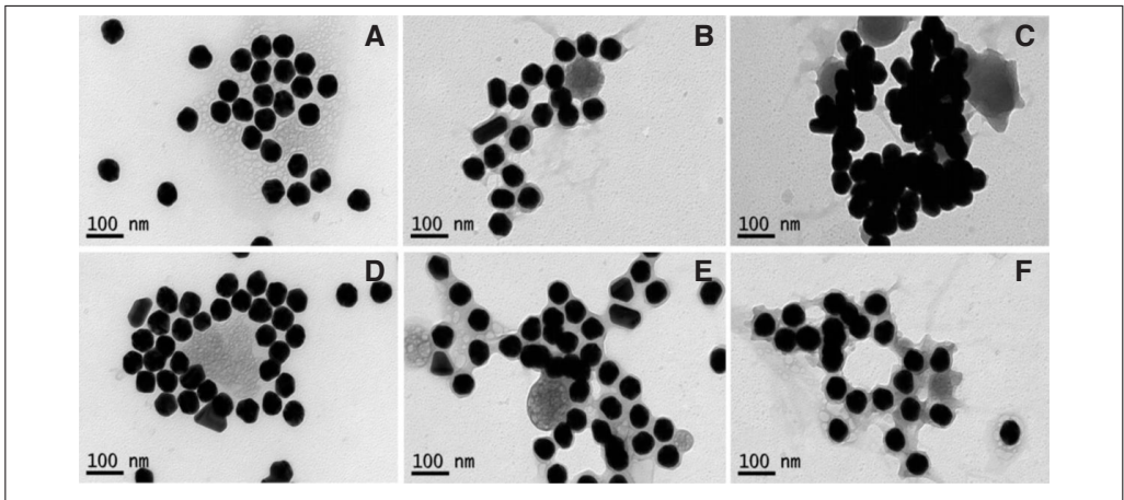
Figura 6. Nanopartículas de oro antes (A) y después de ser esterilizadas mediante radiación ultravioleta (B), gas plasma (C), óxido de etileno (D), formaldehído (E) y autoclave (F).
