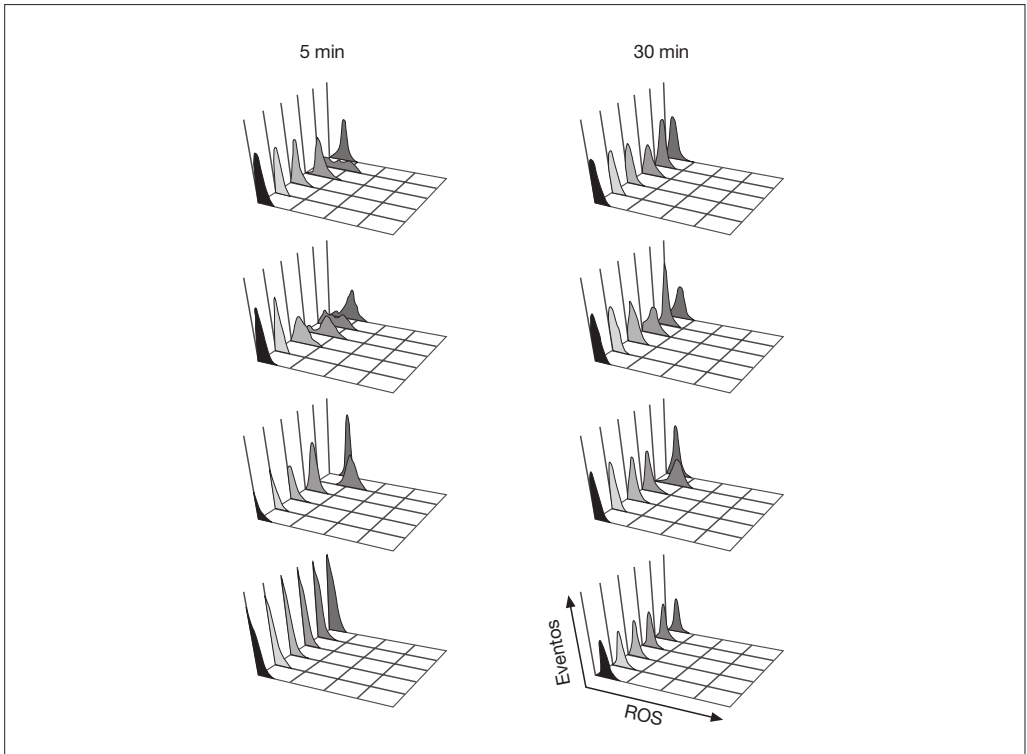
Figura 8. Producción de ROS por parte de distintas células humanas de sangre periférica en presencia de cinco nanopartículas diferentes. Como control negativo se utilizaron células solas (en negro).
