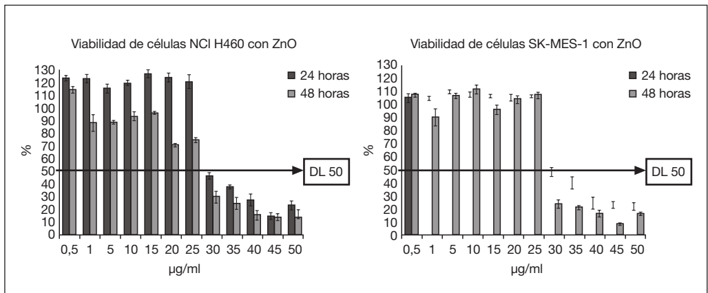
Figura 2. Estudio de muerte celular (dependiente de la dosis) inducida por nanopartículas de zinc en células NCI-H460 y SK-MES.
