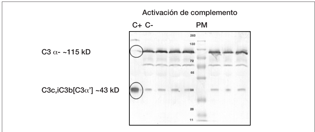
Figura 9. Detección del factor C3 y de productos de degradación mediante Western blot de plasma humano en ausencia (C-) o presencia de nanopartículas. Como control positivo (C+) se empleó veneno de serpiente.
